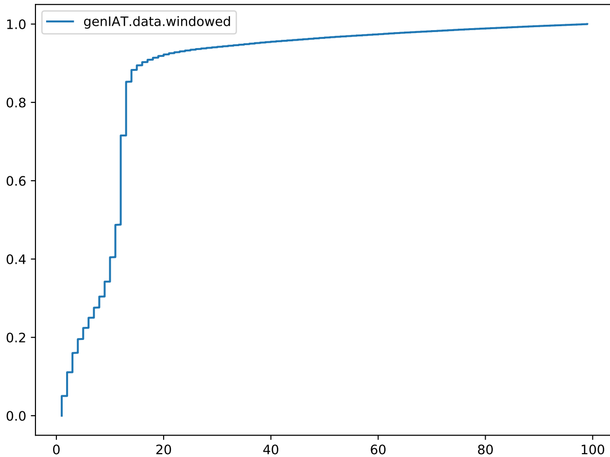
[ ] general - genIAT.data.windowed
